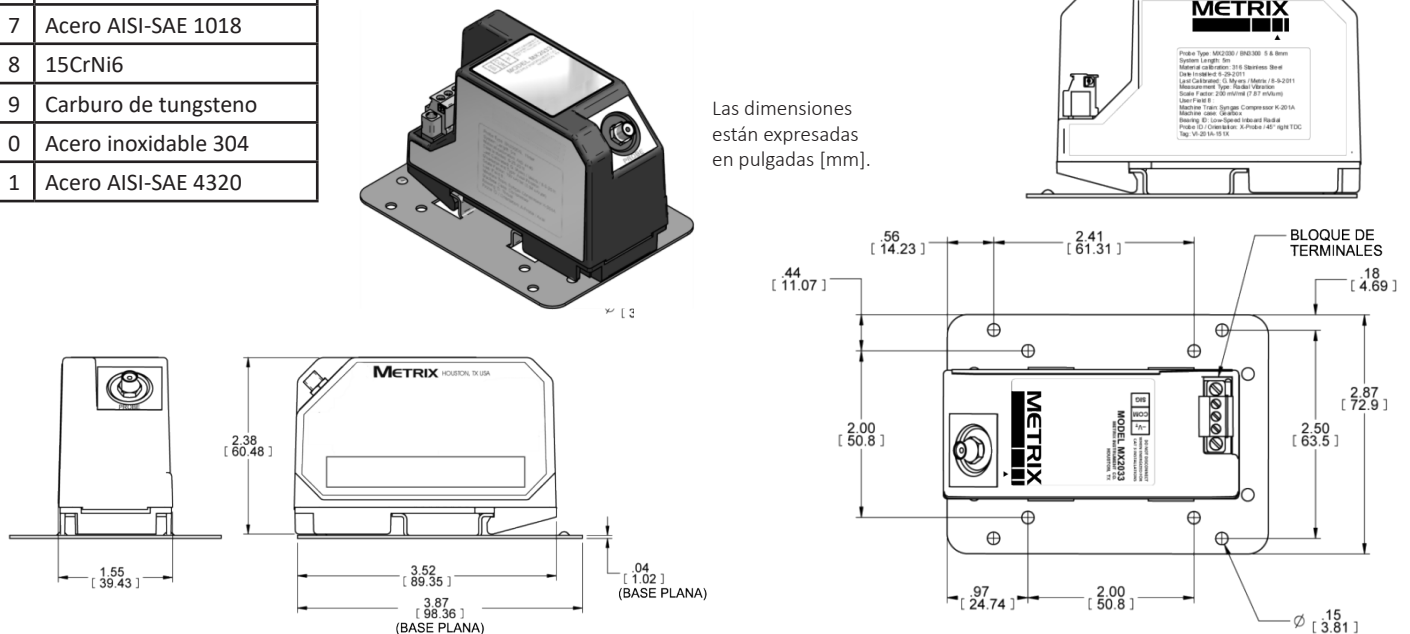
Figura 1: Dimensiones en pulgadas [mm] para el controlador de proximidad digital de 3 hilos MX2033 Nota: se muestra el adaptador de montaje opcional de la placa base de 4 agujeros (N/P 9647). El montaje de riel DIN de 35 mm es estándar.
