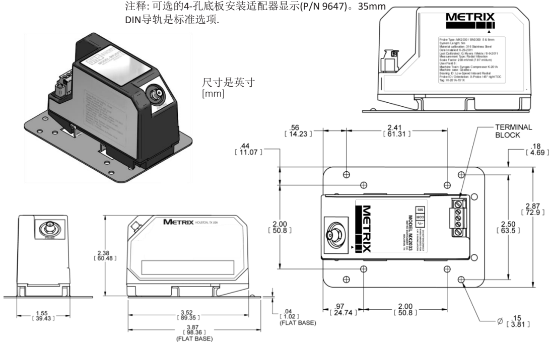
图1: 尺寸为英寸 [mm] 对于MX2033 3-线制数字趋近式前置器。
